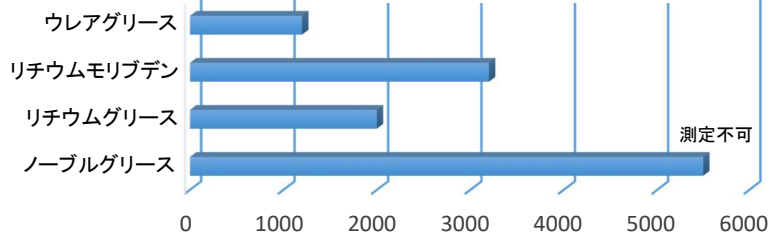
塩水噴霧試験 JIS K2246
