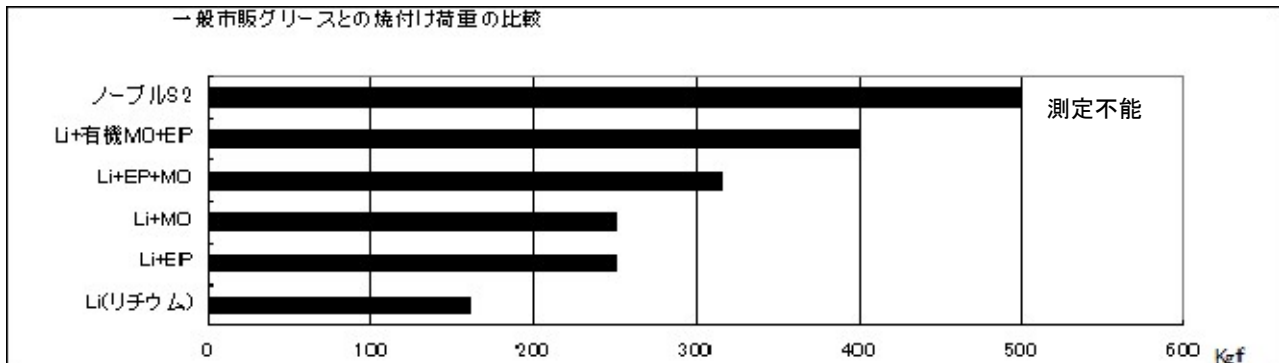
一般市販グリースとの焼付け荷重の比較
